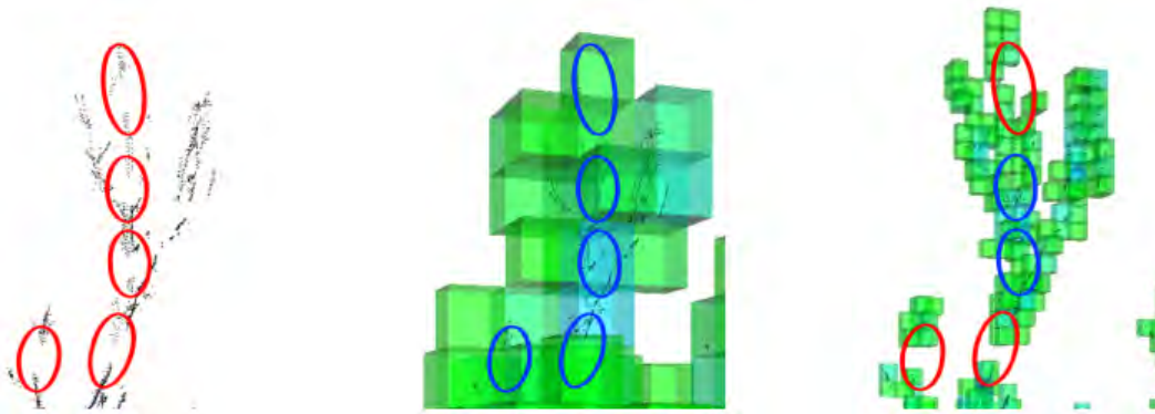
Figure 1.10 Le nuage de point LiDAR d'une branche isolée (à droite), au centre ce même nuage de points voxelisé à une résolution de 0.2 m et à droite à 0.05 m. Les ellipses rouges représentent des zones d'occlusion et les ellipses bleues ces mêmes zones d'occlusion compensées par la voxelisation.
