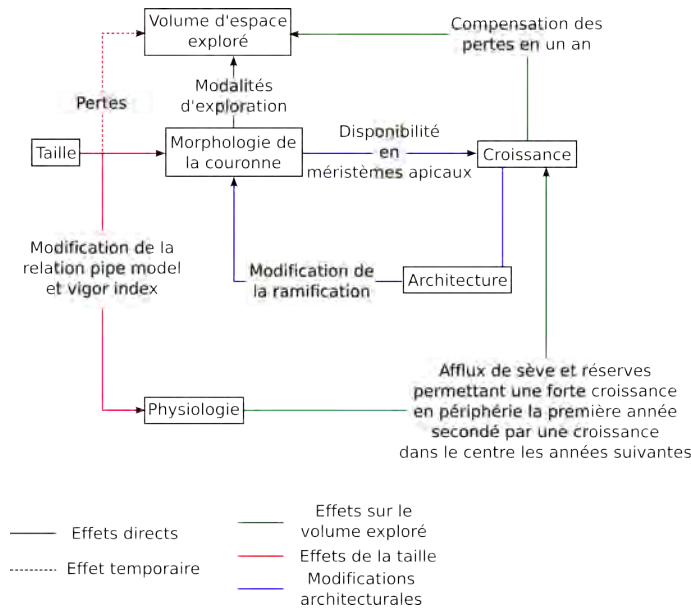
Figure 2.7 Schéma de synthèse du système arbres / tailles unidirectionnelles en V. La légende est indiquée dans le graphique.
