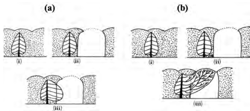
Figure 0.1 Schéma proposé par Hallé (1986) illustrant l'adaptation aux modifications de condition lumineuse de l'environnement par réitération adaptative. (a) : un arbre unitaire dépourvu de la capacité de réitération; (b) : un arbre coloniale capable de réitérer. (i) l'arbre dans son environnement initial, (ii) une trouée apparaît à proximité de l'arbre, (iii) l'arbre réagit.
