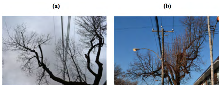
Figure 0.2 Photographies illustrant la mise en place de réitérations traumatiques suite à des tailles intensives. (a) photographie de réitérations traumatiques sur un Frêne d'Amérique ( Fraxinus americana ); (b) prolifération de réitérations traumatiques sur un Érable argenté ( Acer saccharinum ).
