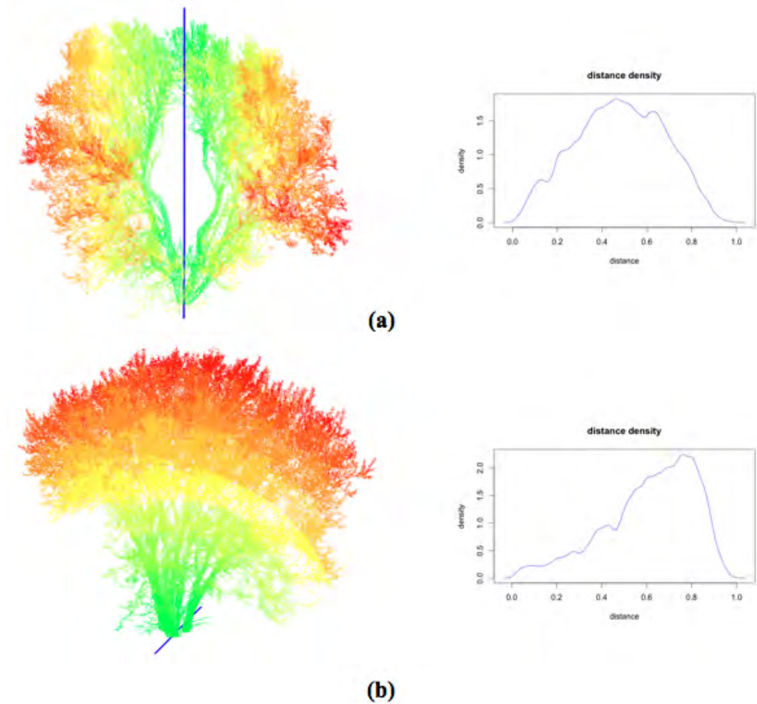
Figure 1.3 Exemples d'utilisation de la fonction « axis.distance.dispersion ». (a) l'axe de référence est l'axe des z. (b) l'axe de référence est l'axe des y. L'axe de référence est représenté en bleu. Pour (a) et (b) les graphiques de densité des distances sont tracés à droite.
