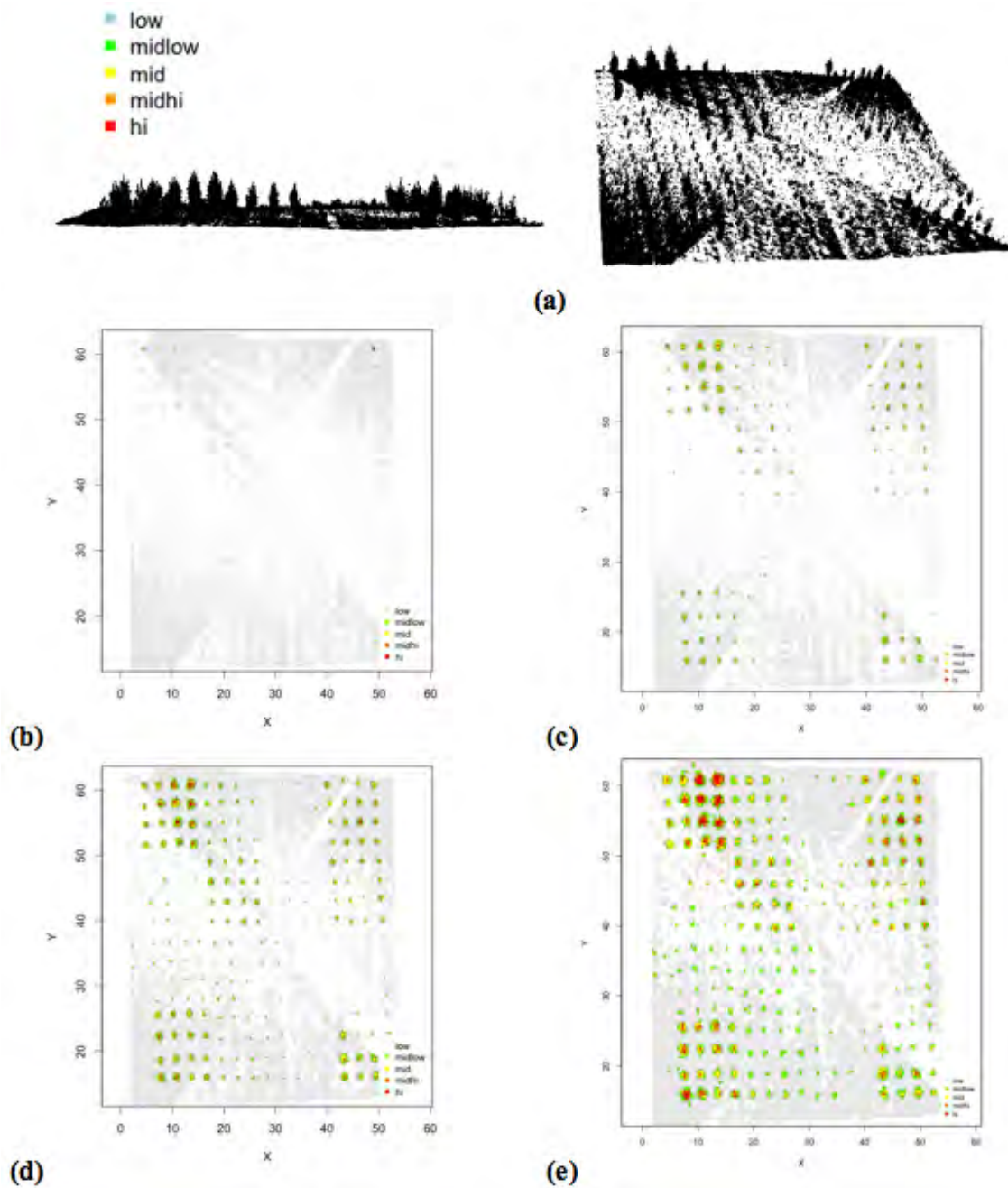
Figure 1.6 Exemples d'utilisation de la fonction « project », visualisée à l'aide de la fonction « raster.projection » pour la projection de la plantation. (a) nuage de points brut, en haut vu de 3/4, en bas vue de face. (b) projection du nombre de points (npts). (c) projection du nombre de voxels (nvox) d'une résolution r = 0.1 . (d) nvox, r = 0.2 . (e) nvox, r = 0.4 . La légende des classes de densité est présentée en haut à gauche.
