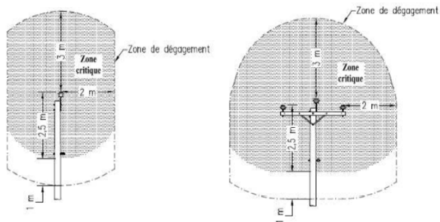
Figure 0.3 Schéma des préconisations de dégagements critiques imposées par Hydro-Québec autour des réseaux électriques. La zone grise représente le volume à l'intérieur duquel aucun élément de végétation ne doit être présent ; à gauche : autour des lignes de distribution basse tension ; à droite : autour des lignes de distribution moyenne tension (Hydro-Quebec, 2009).
