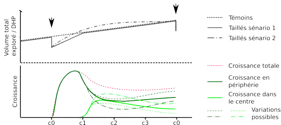
Figure 2.6 Graphiques de synthèse du modèle de croissance théorique prenant part à un cycle de taille. La légende est indiquée dans le graphique.
